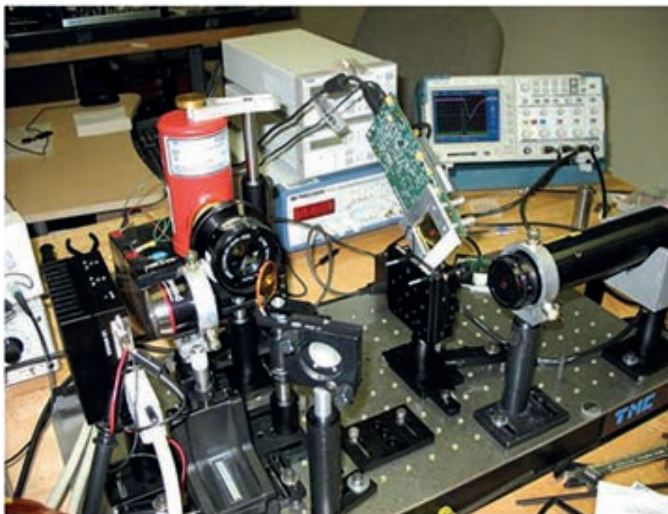
Kvantno-kaskadni laser s digitalnim elektronskim podešavanjem valne duljine (SSI, SAD)
