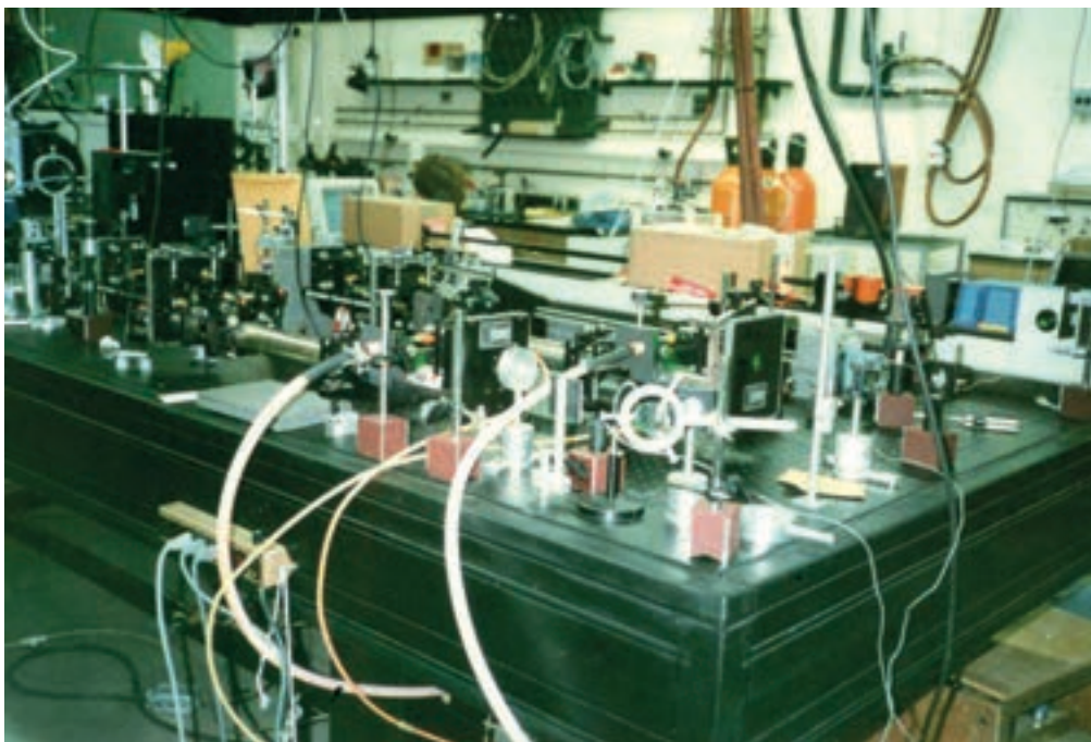
Tečni laser s organskim bojama za spektroskopiju plinova unutar laserskog rezonatora (Sveučilište Arizone, Tucson, SAD)
